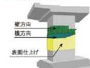
連続繊維シート巻立て工法
