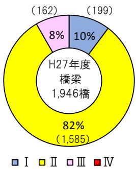
○判定区分と建設経過年度(橋梁)
