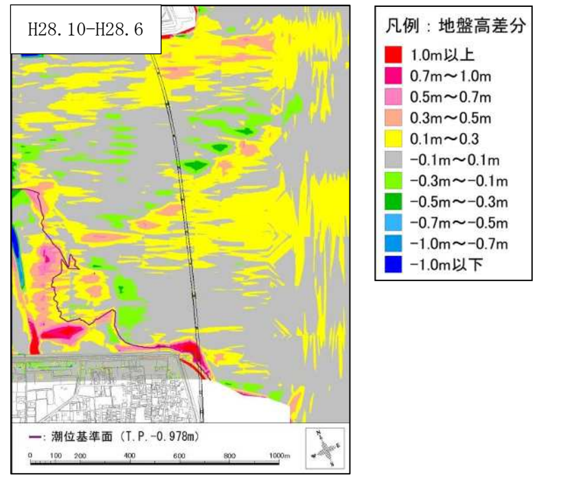
図 4.3-2(4) 橋脚周辺の地形の変遷(平成28年6月～平成28年10月)
