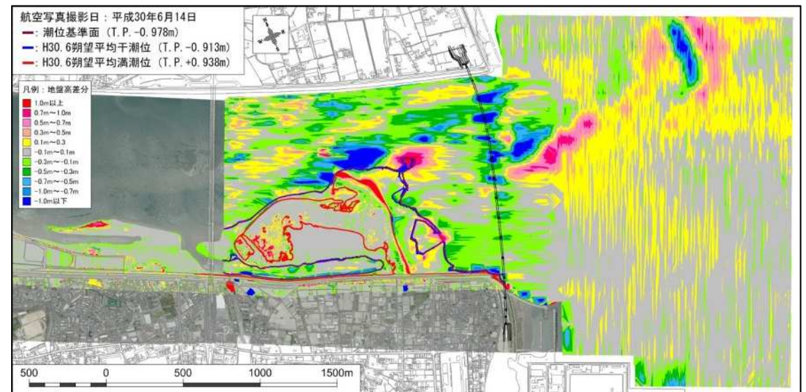
图 4.3-1(8) 平成 30 年 6 月地形調査(水位・降水量、航空写真、地形図、地形差分図(対前回調査))
