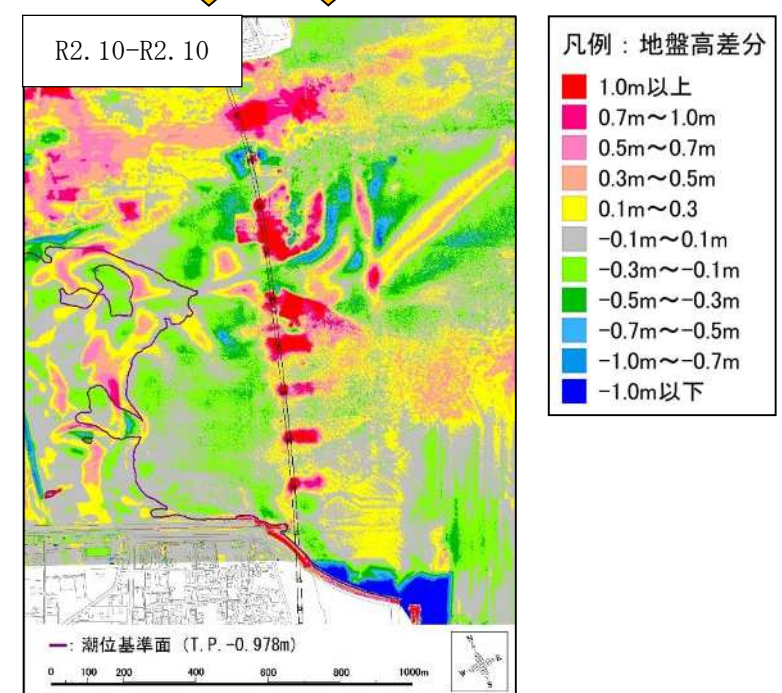
図 4.3-2 (12) 橋脚周辺の地形の変遷(令和2年6月～令和2年10月)
