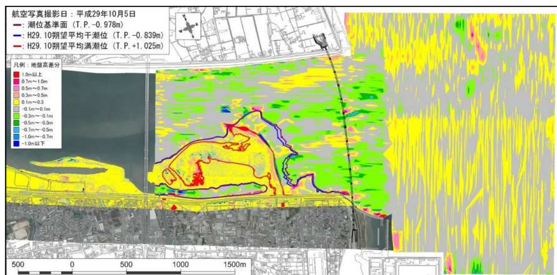
图 4.3-1(7) 平成 29 年 10 月地形調査(水位・降水量、航空写真、地形図、地形差分図(対前回調査))
