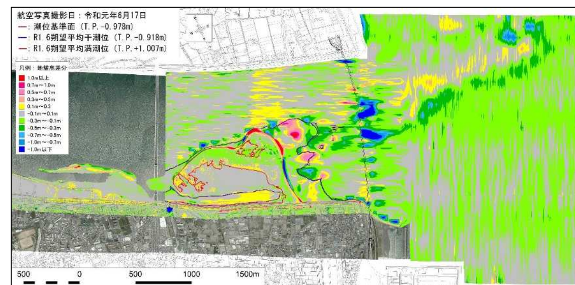
図 4.3-1(10) 令和元年 6 月地形調査(水位・降水量、航空写真、地形図、地形差分図(対前回調査))
