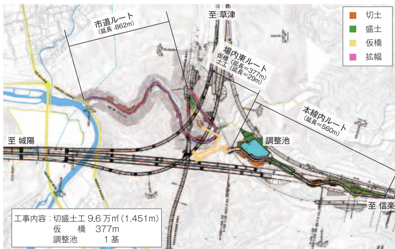
「新名神高速道路 牧工用道路工事」平面図
